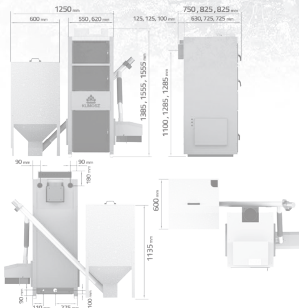
Zmienny wylot czopucha: pionowy / poziomy innowacyjne rozwiązanie opatentowane przez firmę KLIMOSZ
