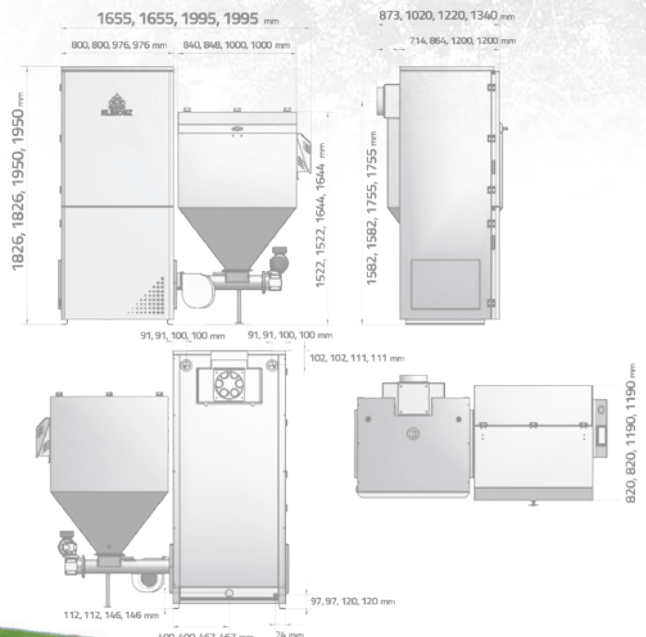
Zmienny wylot czopucha: pionowy / poziomy innowacyjne rozwiązanie opatentowane przez firmę KLIMOSZ
