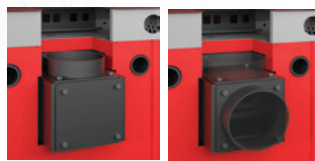
Zmienny wylot czopucha: pionowy / poziomy innowacyjne rozwiązanie opatentowane przez firmę KLIMOSZ
