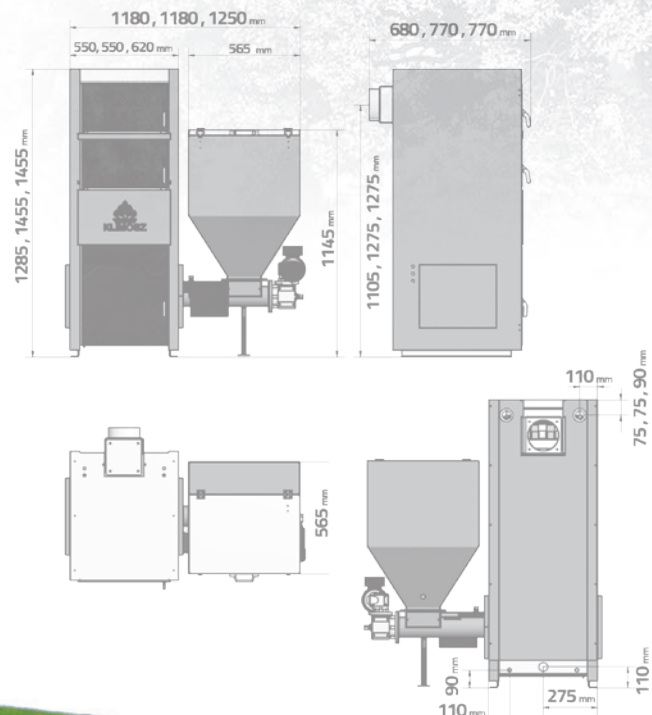
Zmienny wylot czopucha: pionowy / poziomy innowacyjne rozwiązanie opatentowane przez firmę KLIMOSZ
